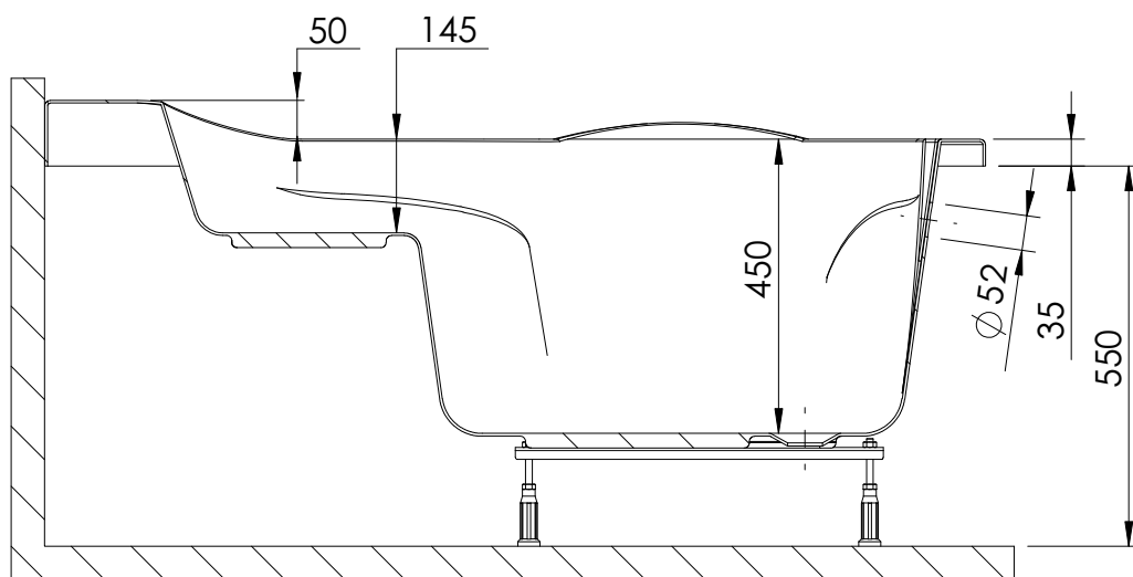
ŘEZ A-A
