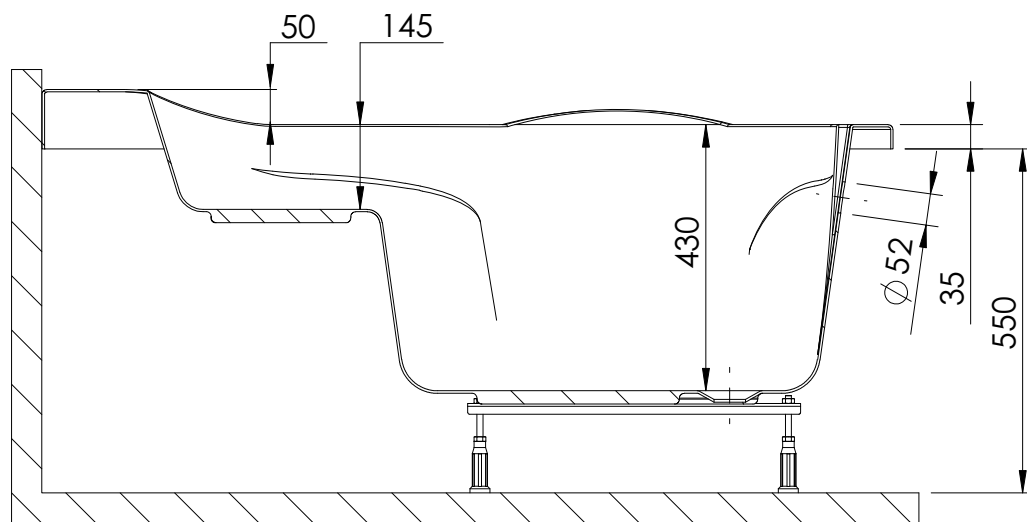
ŘEZ A-A
